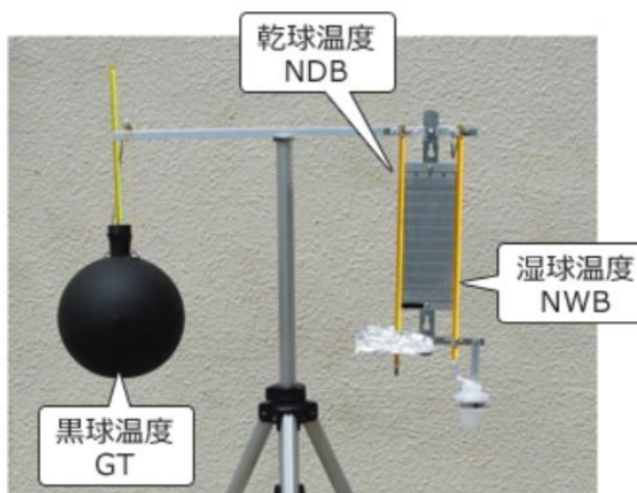
暑さ指数(WBGT)測定装置
