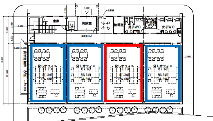
1階平面図
