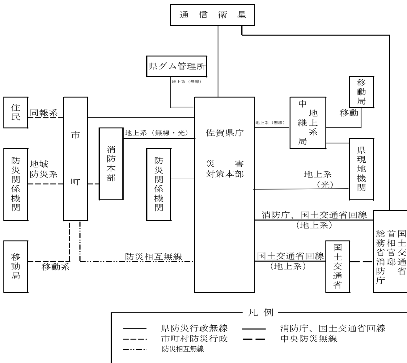
【 通信系統図 】
