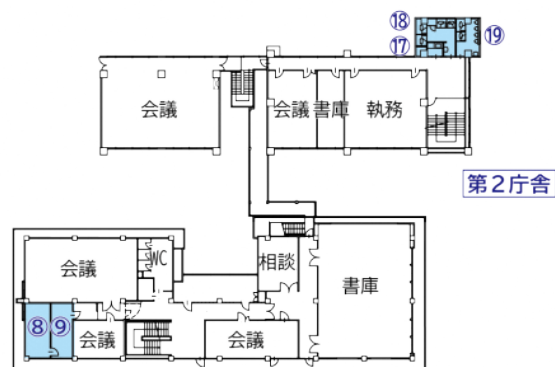
嬉野庁舎3階
