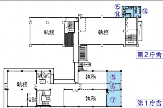
嬉野庁舎2階
