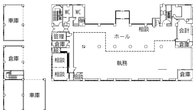
塩田庁舎1階
