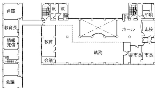
塩田庁舎2階
